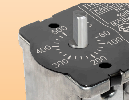
A: 轴直径6mm，长度10mm，用于印刷旋钮和边框，或小塑料箭头旋钮 (可作为下面的配件提供)；
