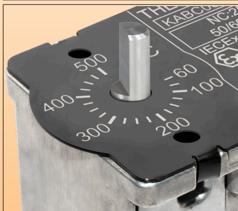
A: 轴直径6mm，长度10mm，用于印刷旋鈕和边框，或小塑料箭头旋鈕 (可作为下面的配件提供)；
