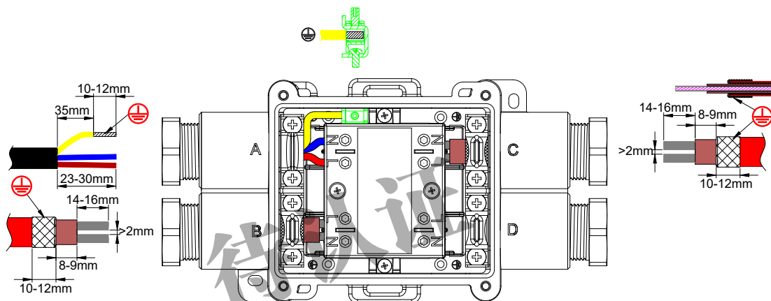
带2根发热线和一根电源电缆的型号
