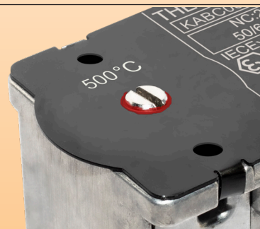
F: 固定的及密封的温度调节
